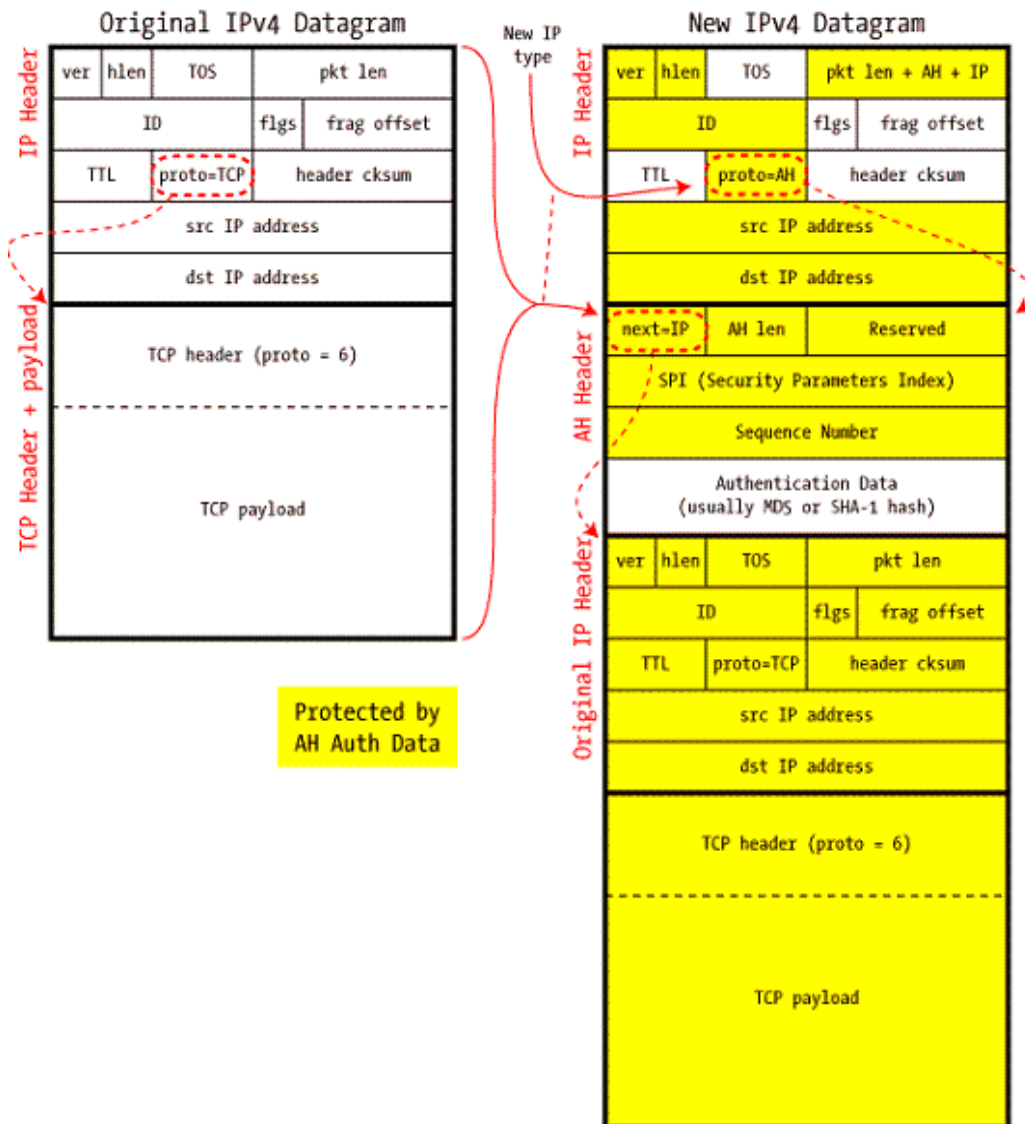
Сурет 2.12 – Туннельді режимдегі АН
