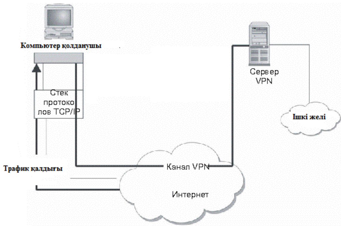
Сурет 2.3 - Ұйымның ішкі желісіне кіру үшін «троя атын» пайдалану
