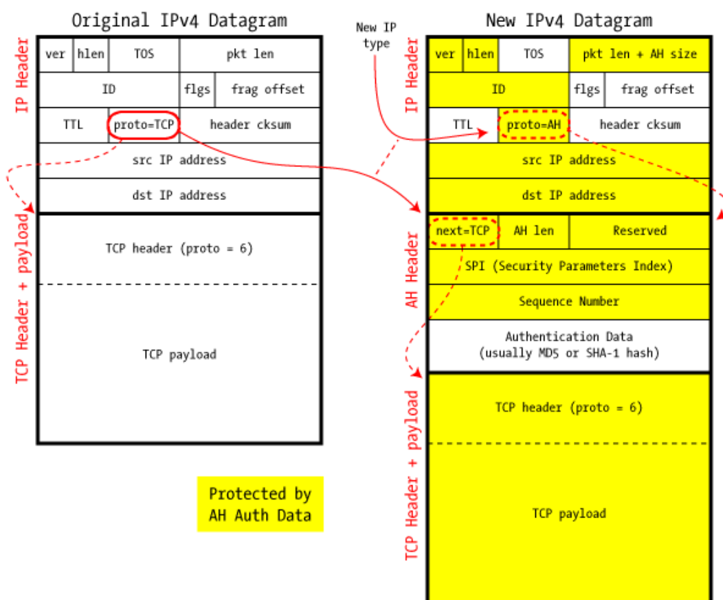
Сурет 2.11 – Тасымалдаушы режимдегі АН
