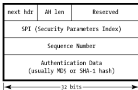
Сурет 2.10 – АН атауының пішіні
