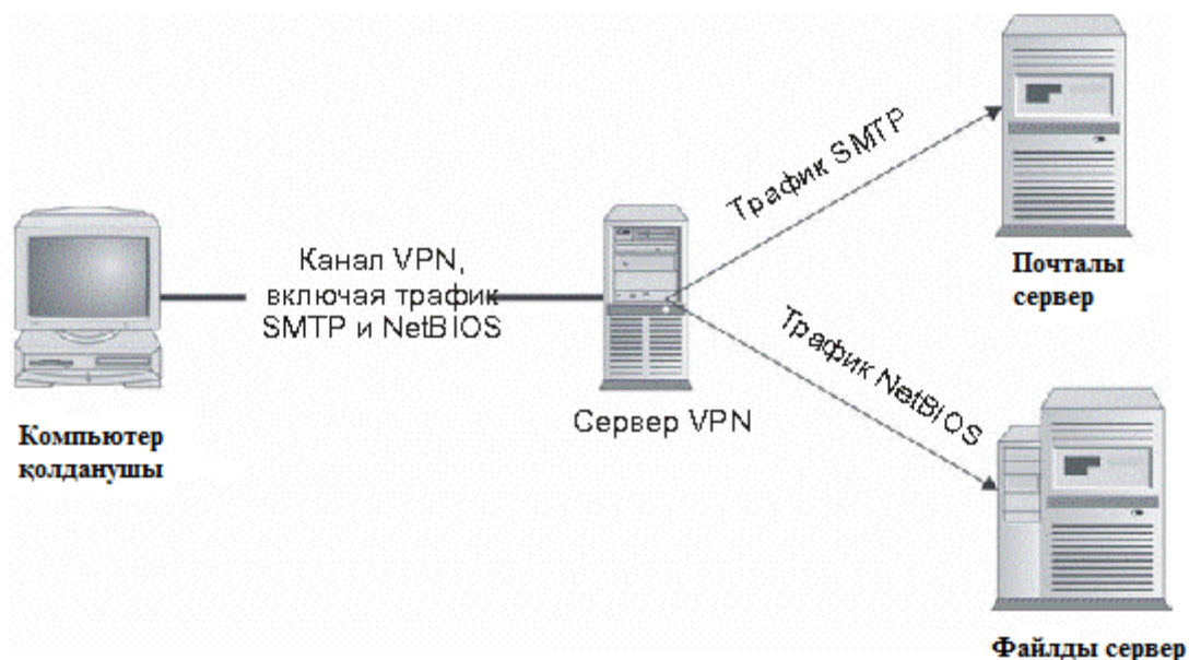
Сурет 2.1 - Виртуалды жеке желілер көптеген хаттамаларға ие
