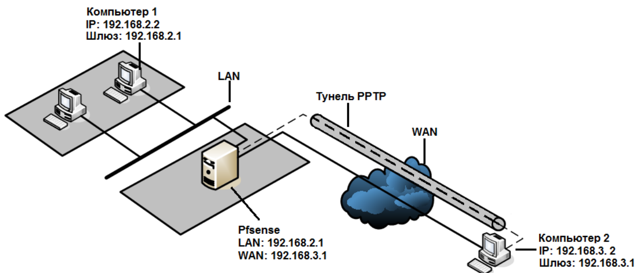
Сурет 3.5 – PPTP хаттамасында туннельді құру
