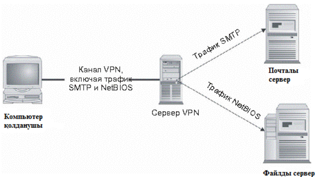
Сурет 1.1 - Виртуалды жеке желілердің хаттамалары
