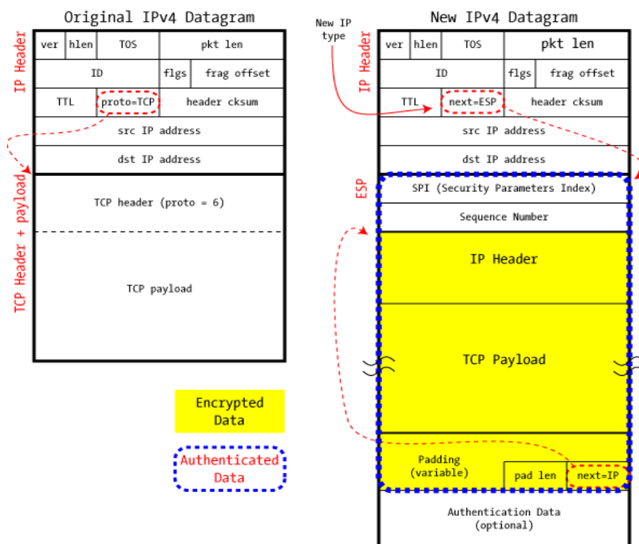
Сурет 3.4 – ESP tunnelmode
