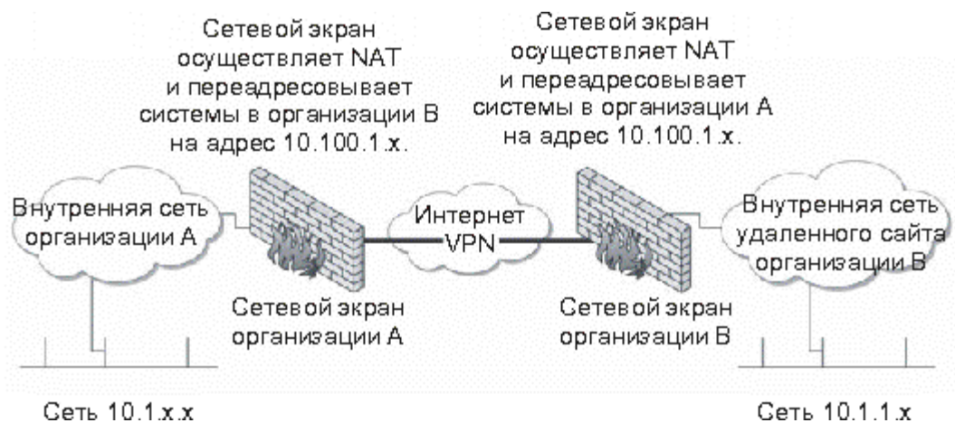
Сурет 2.6 – Тораптық VPN адресстелу келіспеушіліктерінің алдын алу үшін NAT пайдаланады
