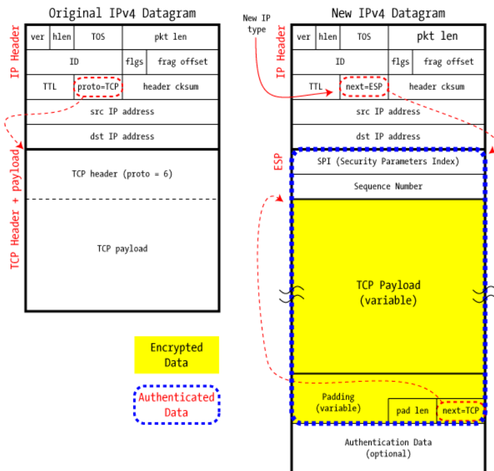
Сурет 3.3 – ESP transport mode
